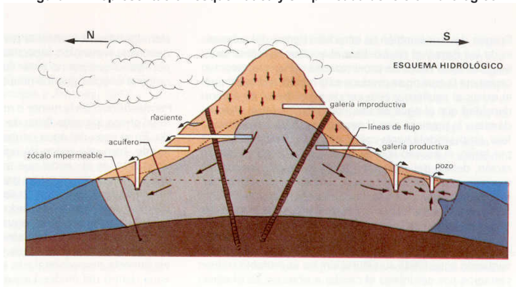
Figura 11. Representación esquemática y simplificada del ciclo hidrológico.
